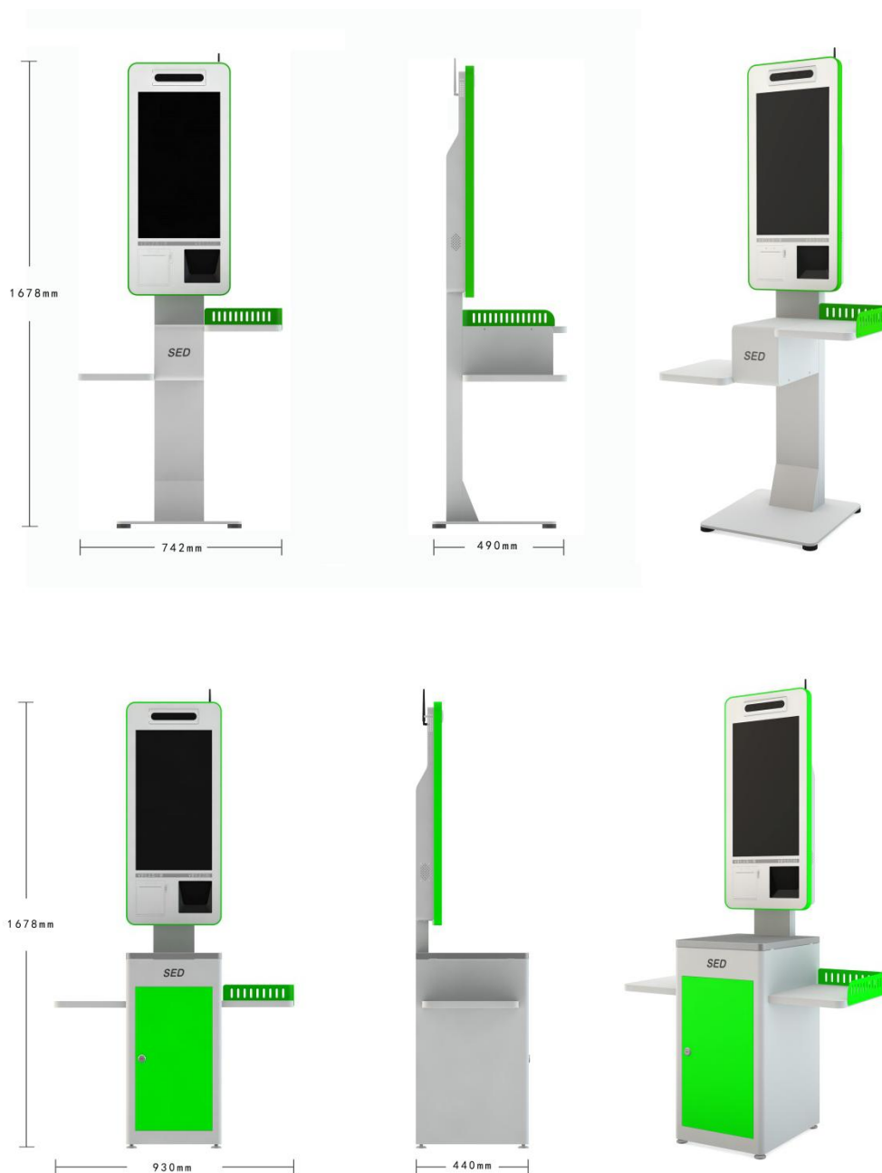
立式支架版本尺寸图
