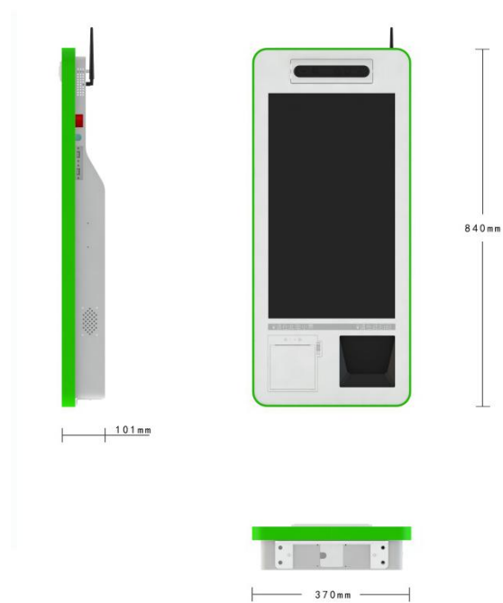
主机尺寸图
