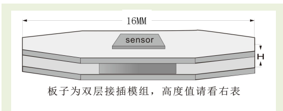
模组高度示意图
